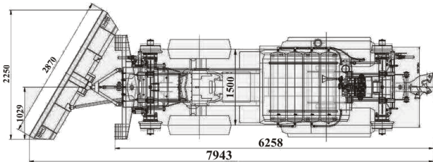
SLIKA 3. DRUMSKO – ŽELEZNIČKI TRAKTOR ZA STANDARDNE I ŠIROKE PRUGE – GORNJI POGLED
