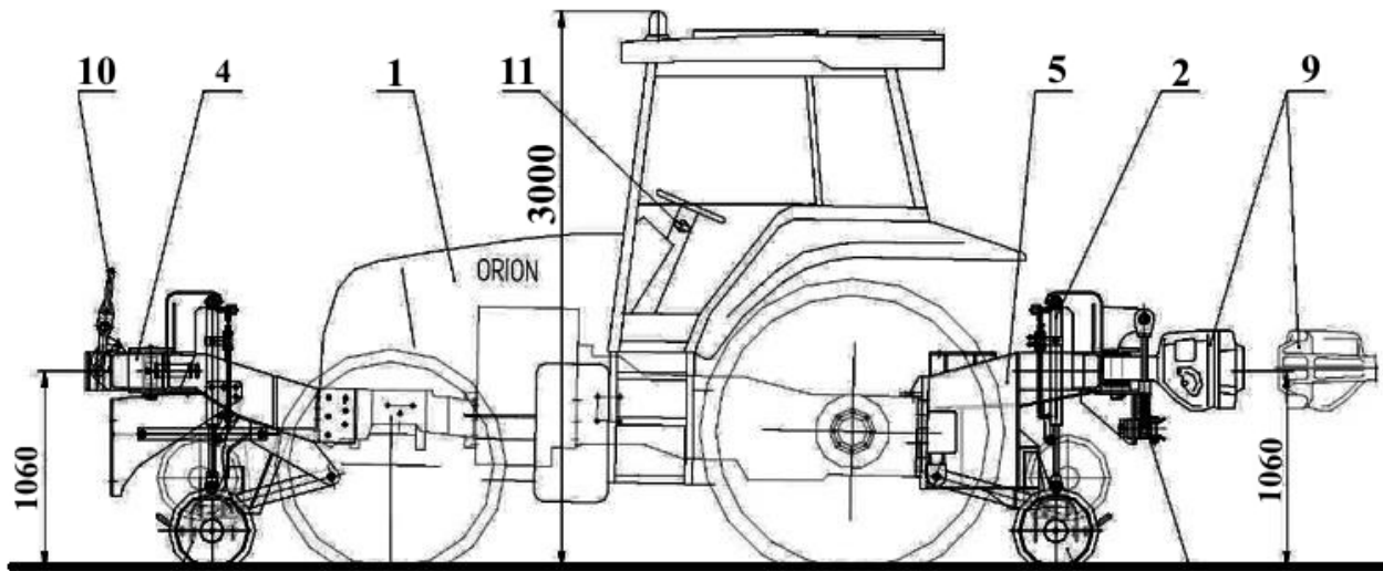
SLIKA 1. DRUMSKO - ŽELEZNIČKI TRAKTOR ZA STANDARDNE I ŠIROKE PRUGE BEZ PNEUMATSKE KOČNICE
