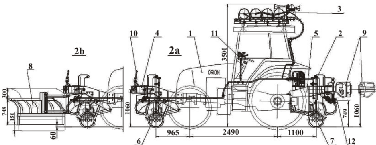
SLIKA 2.a i 2.b DRUMSKO - ŽELEZNIČKI TRAKTOR ZA STANDARDNE I ŠIROKE PRUGE SA PNEUMATSKOM KOČNICOM I PLUGOM ZA ČIŠĆENJE SNEGA
